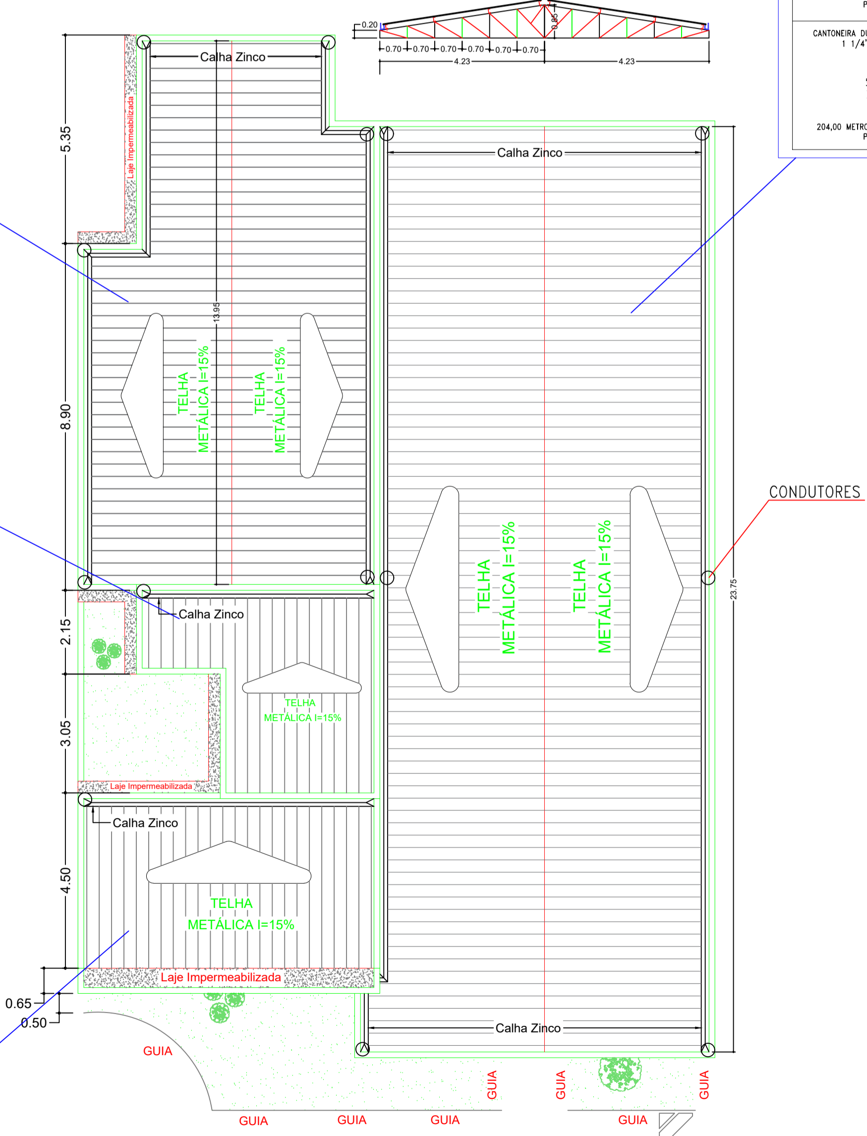
DETALHAMENTO COBERTURA ESCALA 1/100
