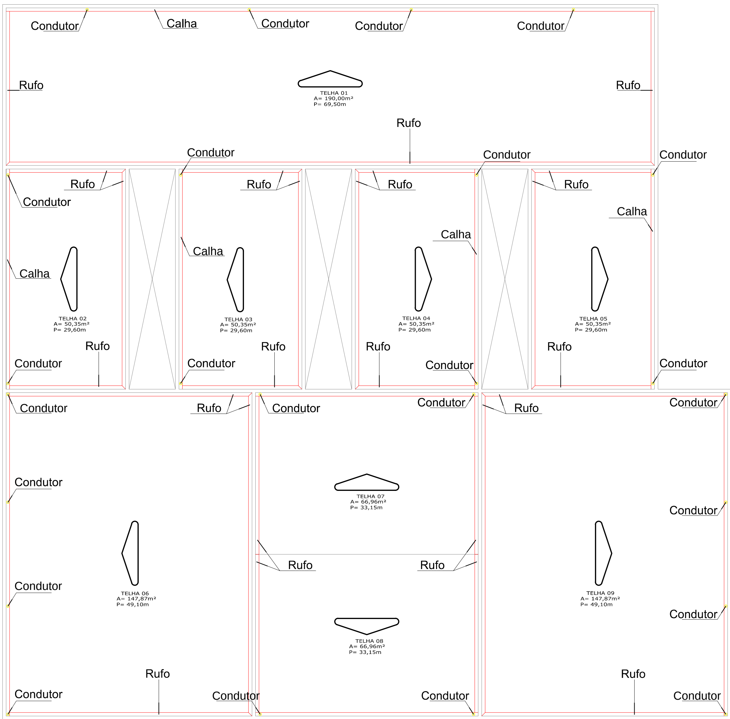
PLANTA DA COBERTURA
