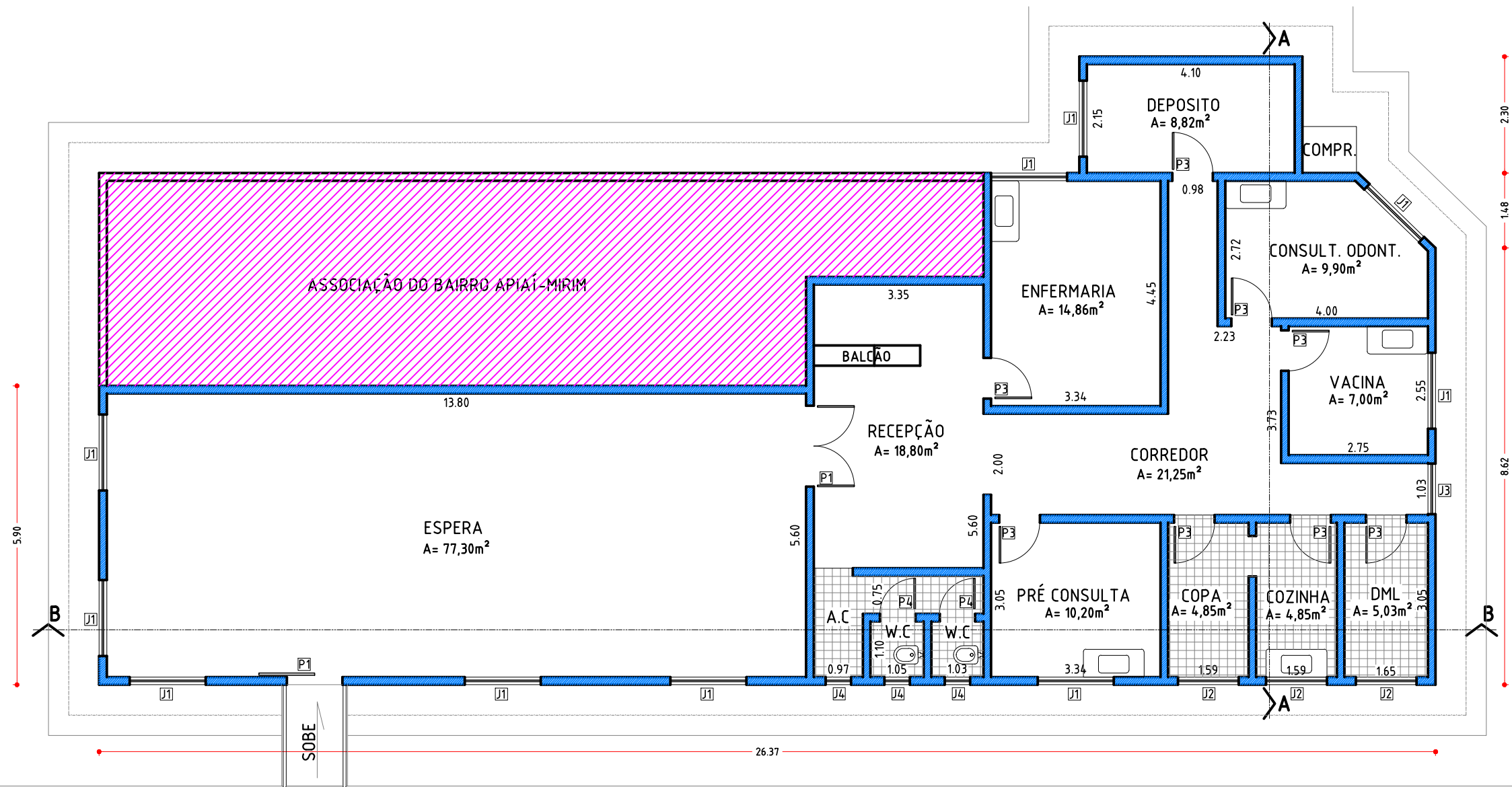
SITUAÇÃO PRETENDIDA ESCALA 1/100
