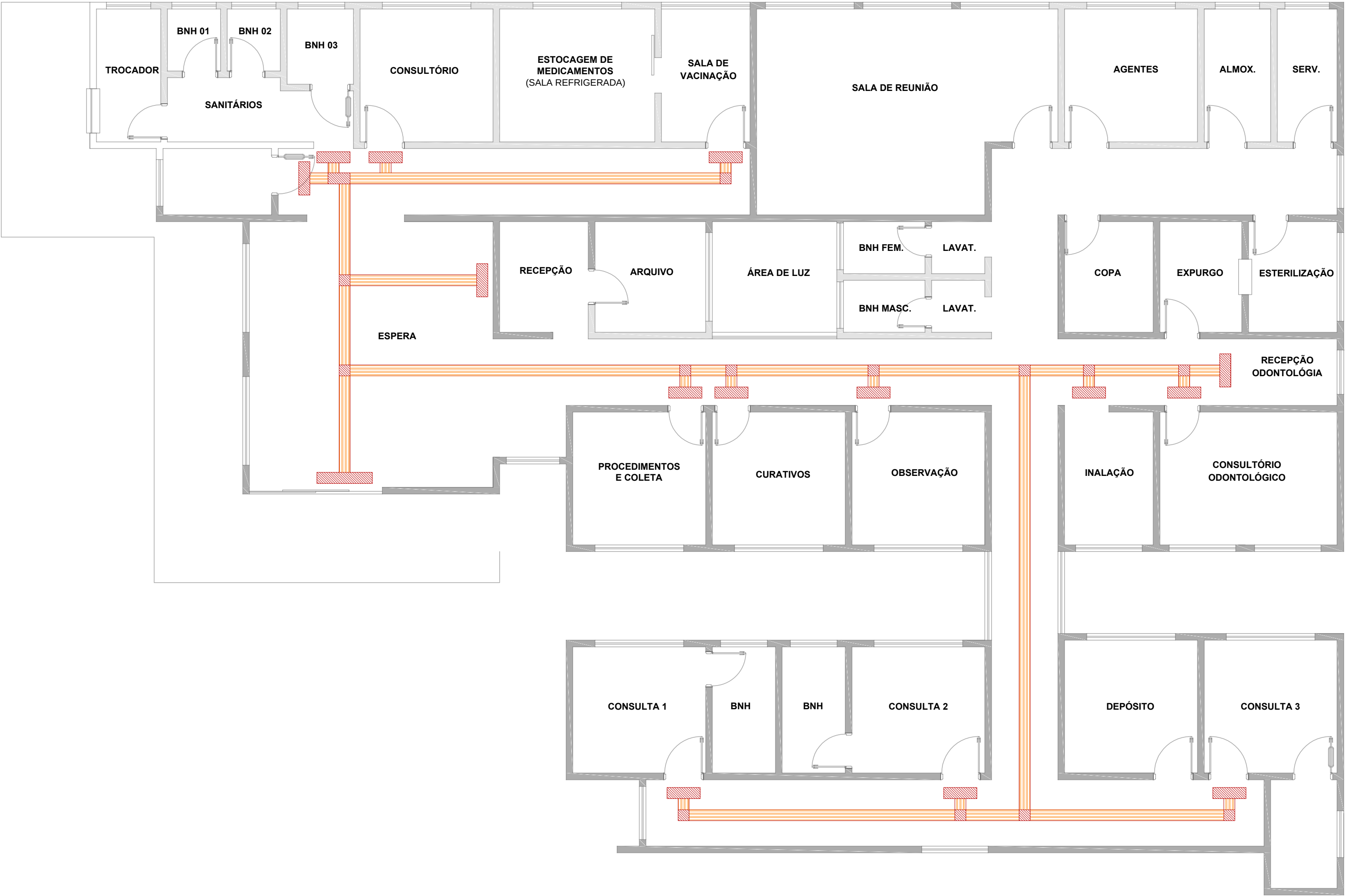
PLANTA BAIXA DE ACESSIBILIDADE – PISO TÁTIL Esc.: 1/75
