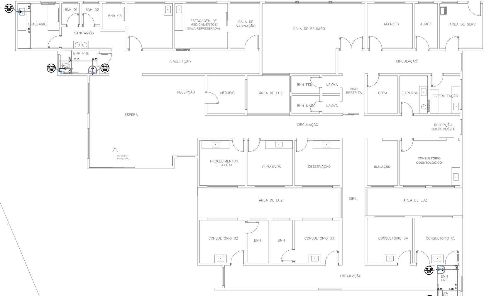
HIDROSSANITARIO ESCALA 1:100
