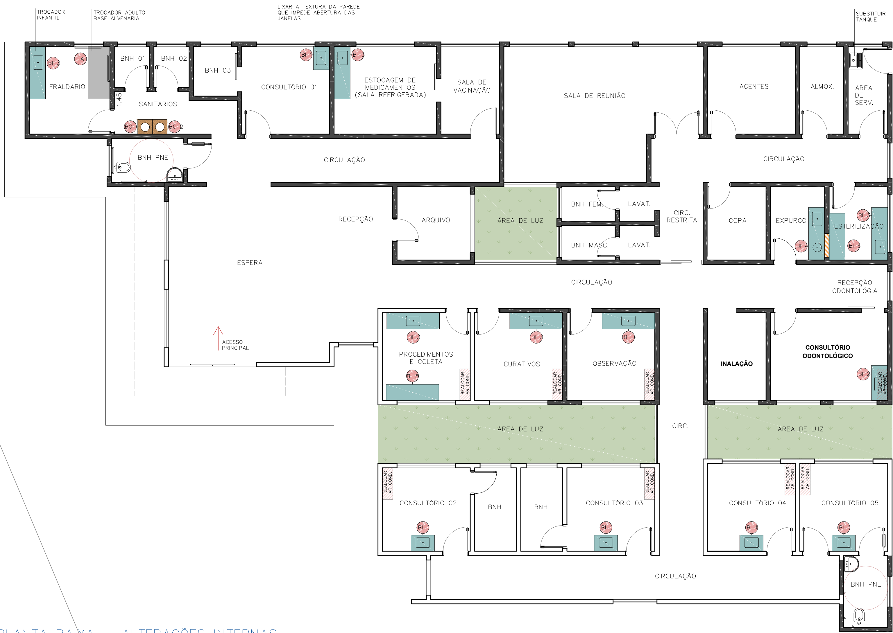
PLANTA BAIXA – ALTERAÇÕES INTERNAS Esc.: 1/75
