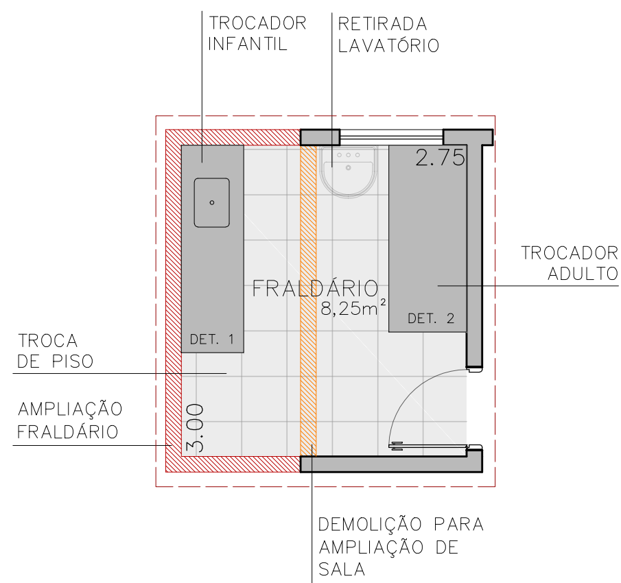
DETALHAMENTO FRALDÁRIO Esc.: 1/50
