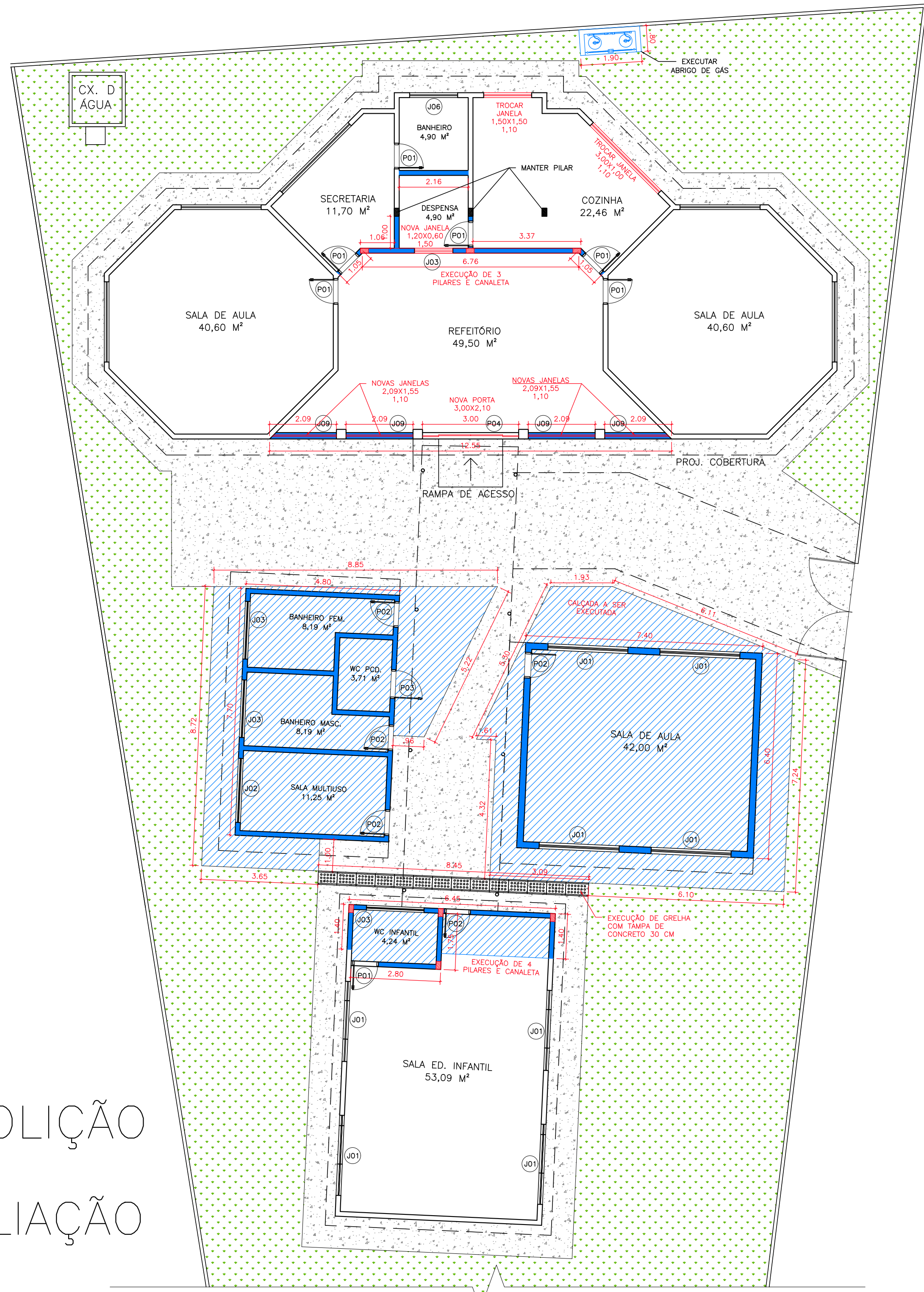
2 SITUAÇÃO PROPOSTA – AMPLIAÇÃO 1:100
