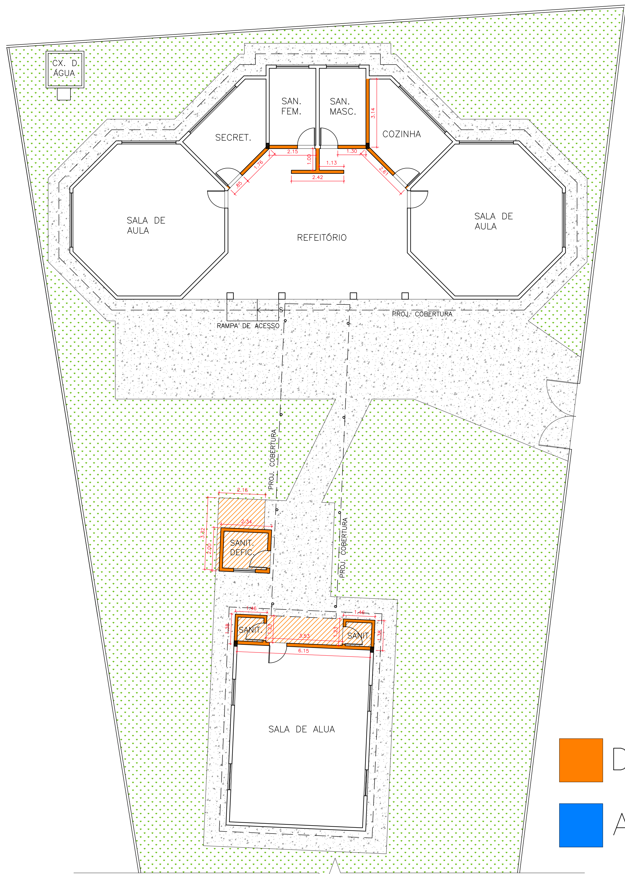
1 SITUAÇÃO ATUAL – DEMOLIÇÃO 1:100
