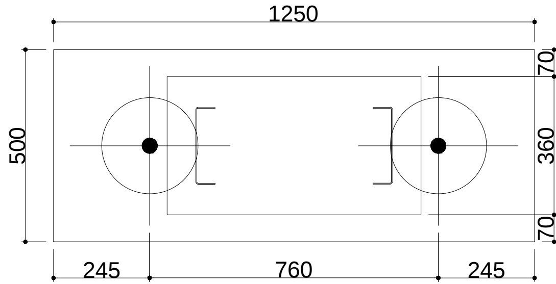
Detalhe dos pilares e placa de base nos blocos escala 1:10
