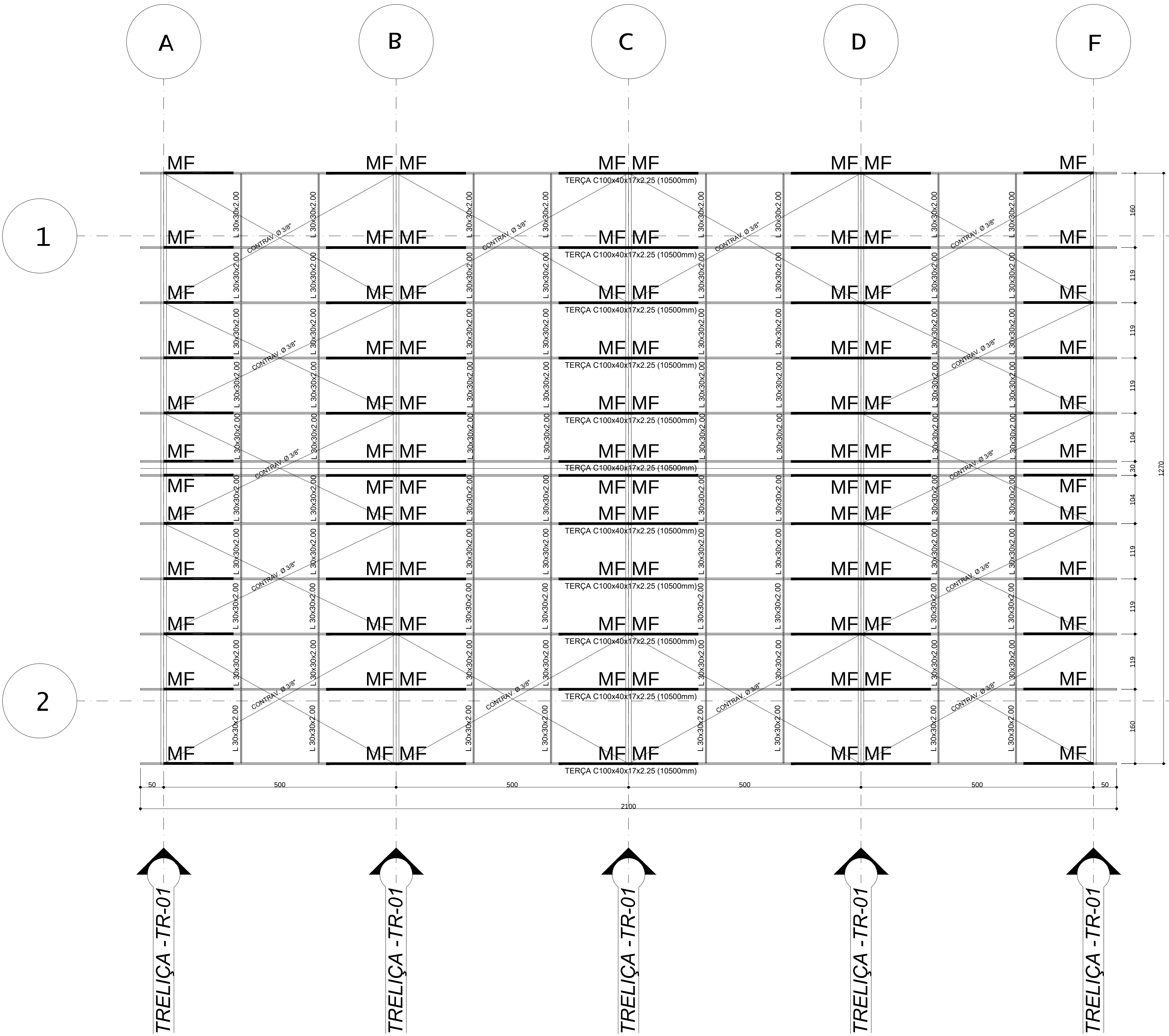
Planta de locação das Placas de base escala 1:50
