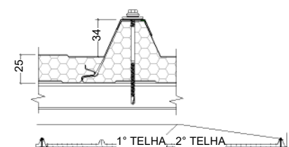
3 DET. 04 - FIXAÇÃO SEM ESCALA
