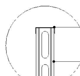
4 DET. 05 - TOPO DE ACAB. DE PAREDE EXPOSTA 1:10
