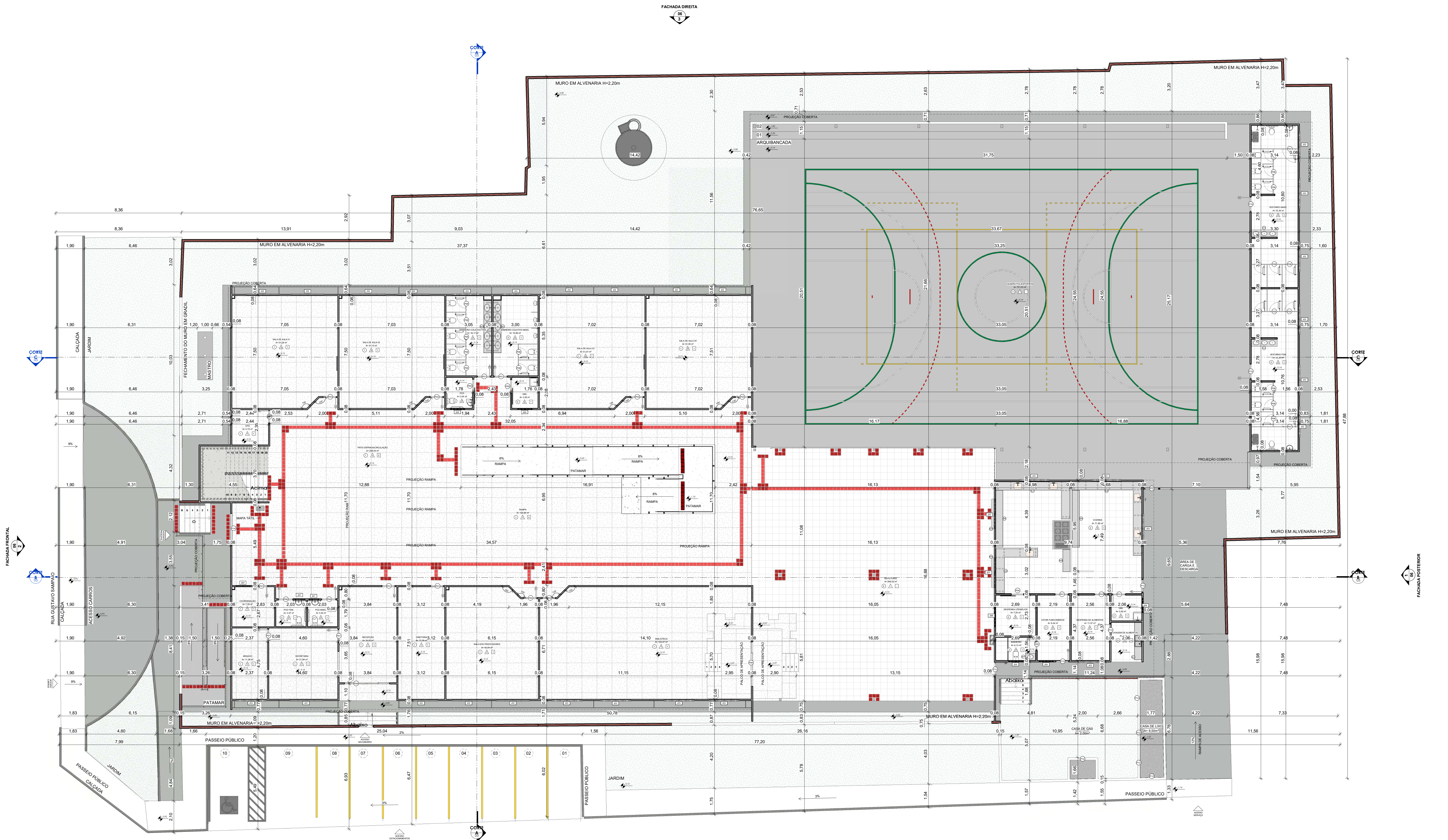
1 PLANTA BAIXA - TÉRREO 1:100
