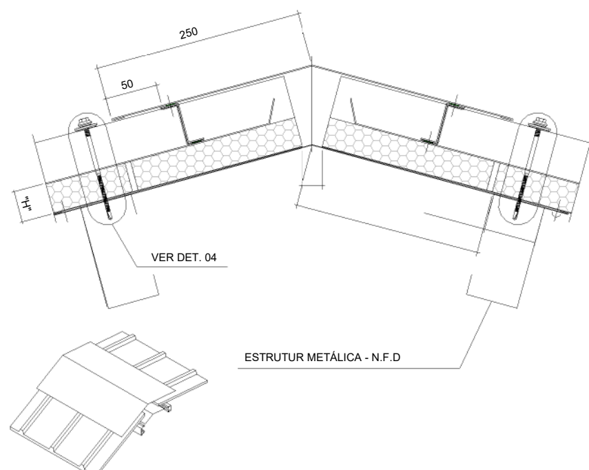
2 DET. 03 - CUMEIRA SEM ESCALA
