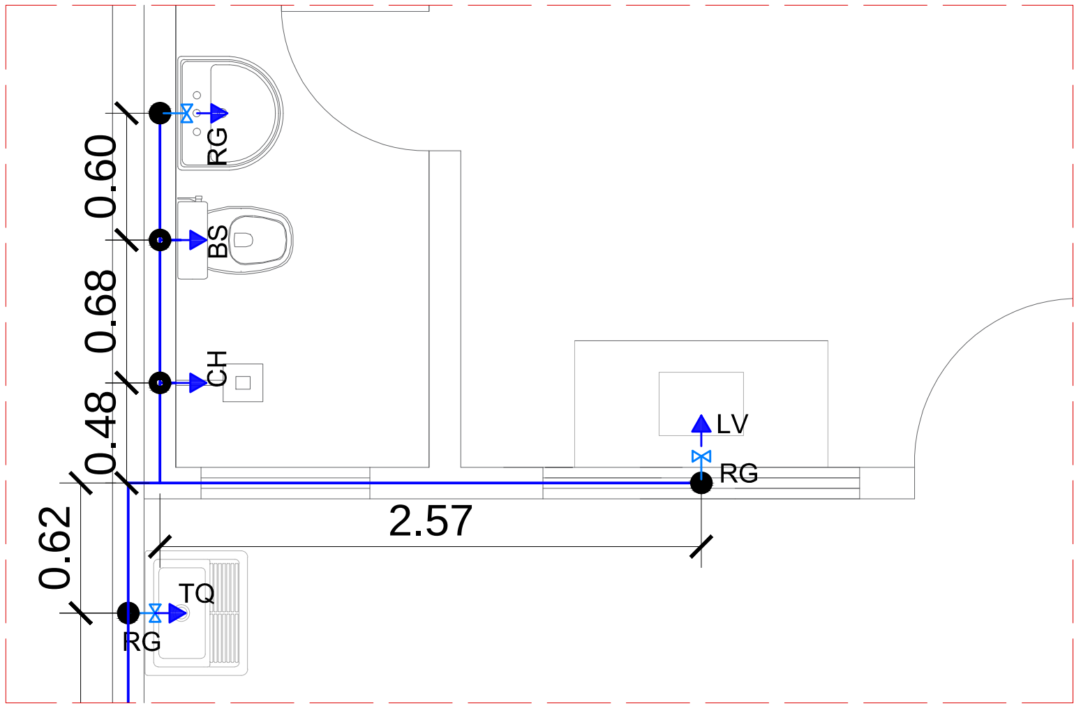
DET. HIDRAULICO Esc.: 1/25
