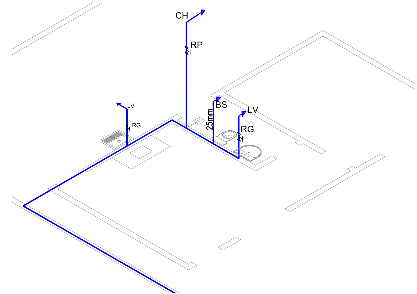
ISOMÉTRICA
