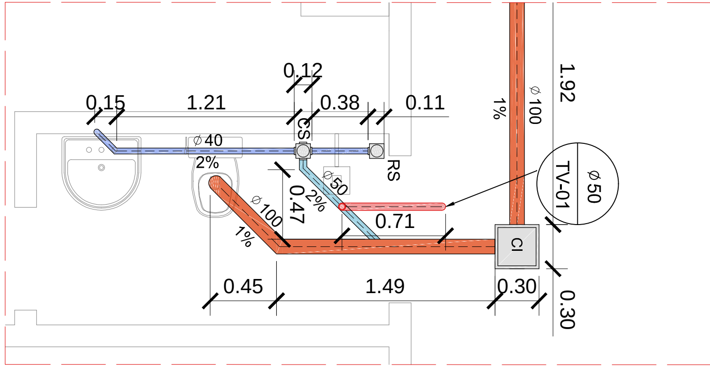
DET. HIDROSANITÁRIO - BANHEIRO Esc.: 1/25
