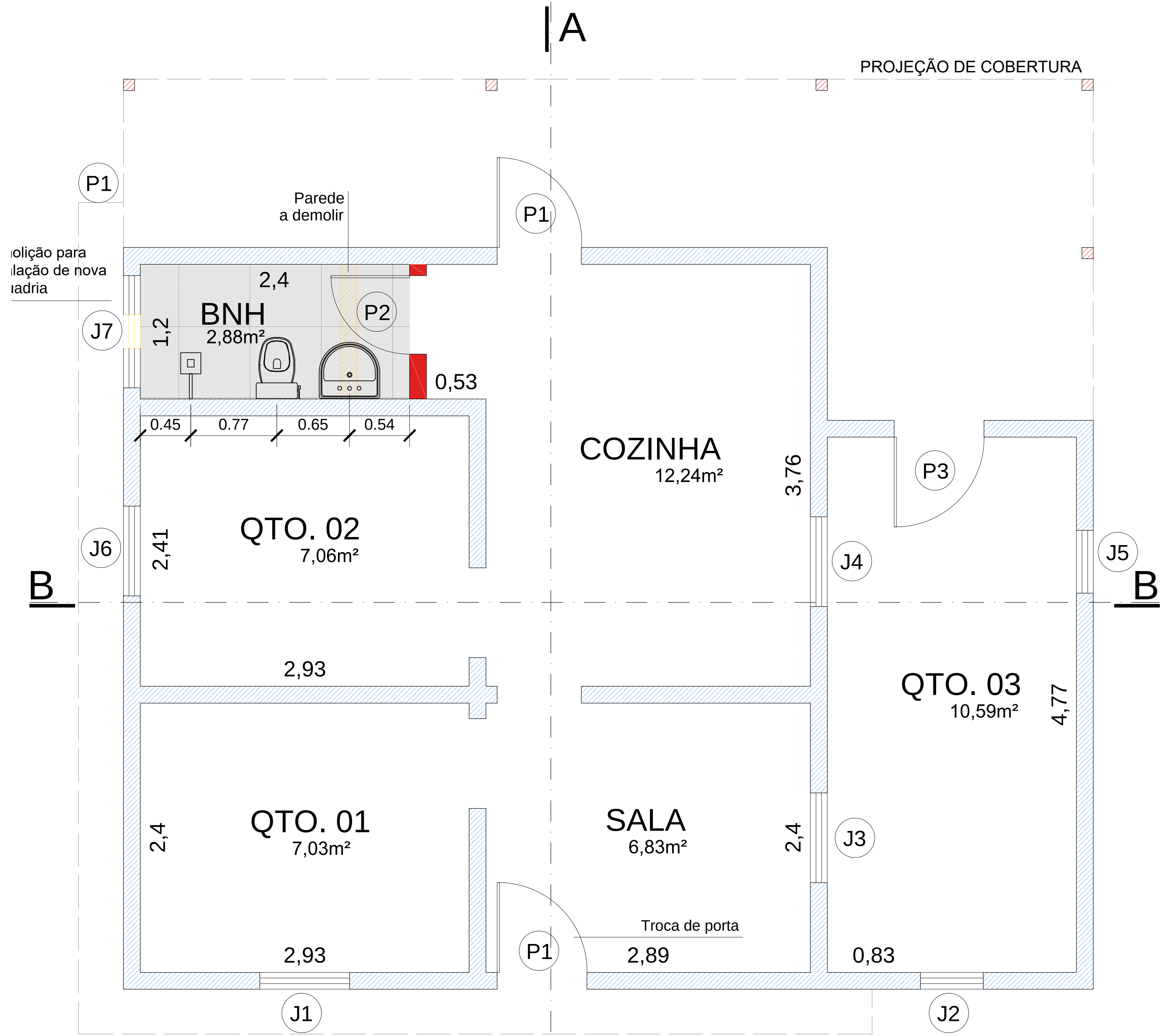
PLANTA BAIXA Esc.: 1/50
