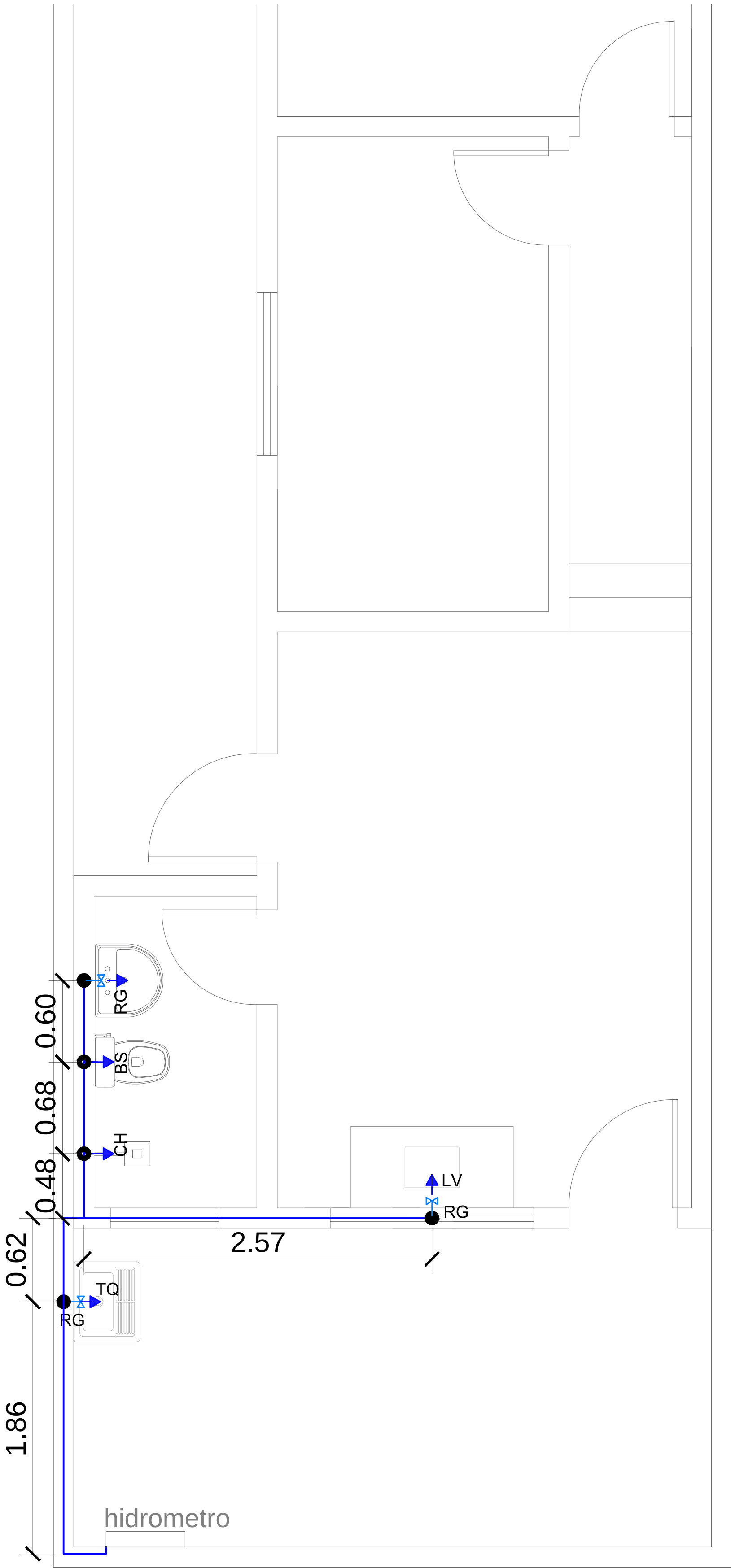
PROJETO HIDRAULICO Esc.: 1/50
