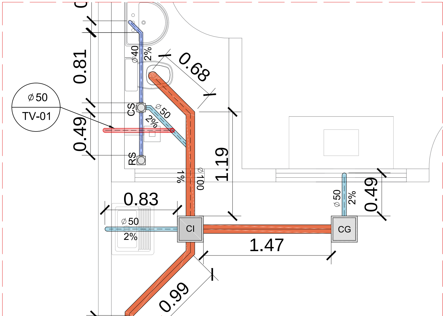
DET. HIDROSANITÁRIO Esc.: 1/25
