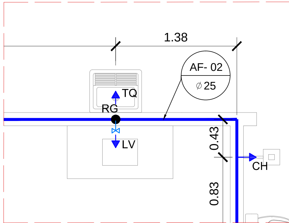
DET. HIDROSANITÁRIO - COZINHA Esc.: 1/25
