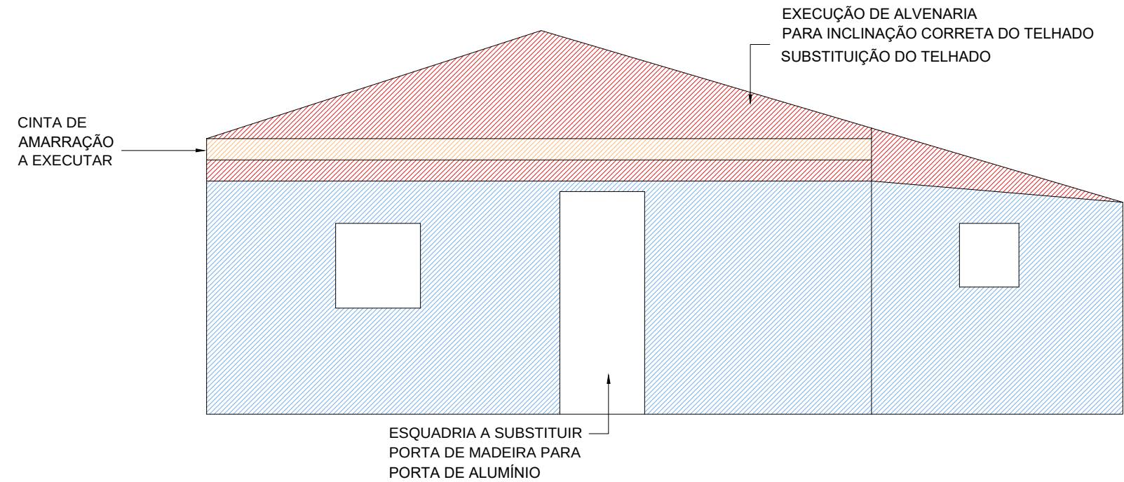
FACHADA PRINCIPAL Esc.: 1/50
