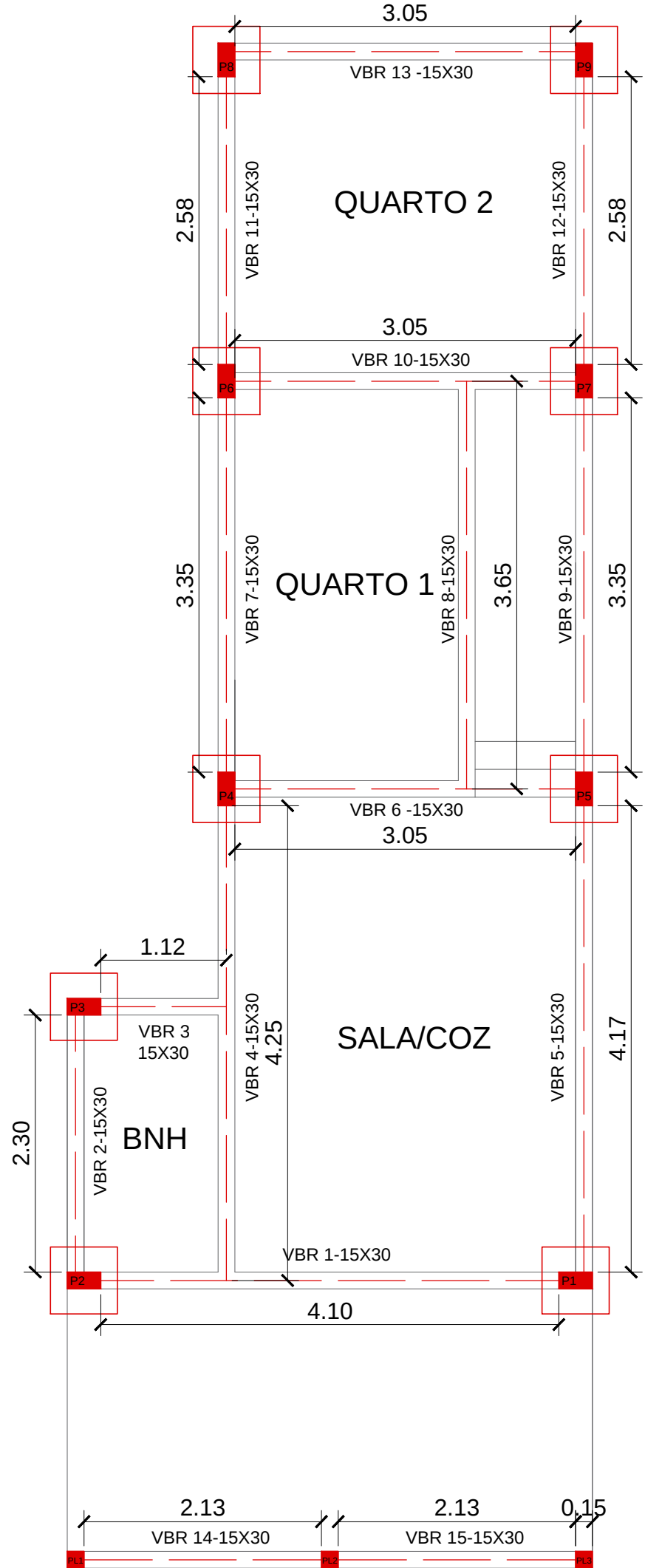
PROJETO ESTRUTURAL - VIGA BALDRAME/PILAR Esc.: 1/50
