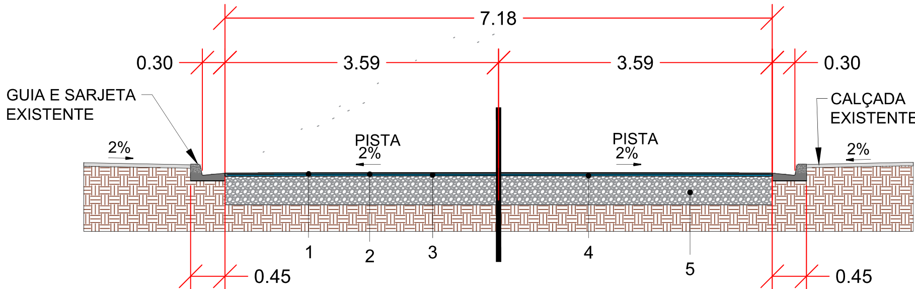
CORTE TRANSVERSAL A-A RECAPEMANETO ASFÁLTICO COM CBUQ AVENIDA DR. TADEU ZAGLOBINSKI VENTURELLI ESC. 1:50
