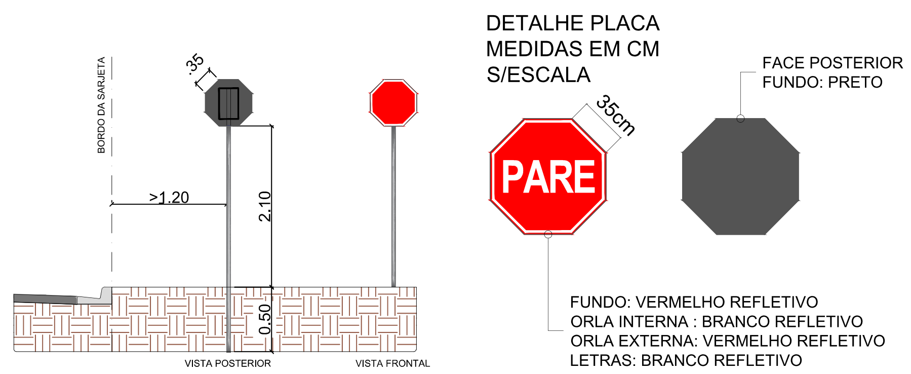
DETALHE PLACA R-1 PARE PLACA - ELEVÇÃO MEDIDAS EM M S/ESCALA
