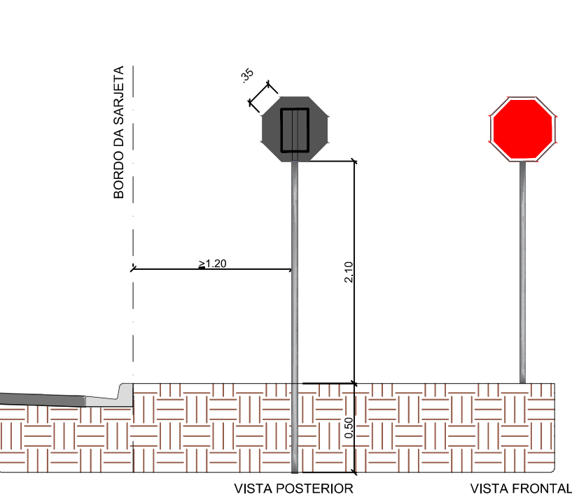
DETALHE PLACA R-1 PARE PLACA - ELEVACÃO MEDIDAS EM M S/ESCALA
