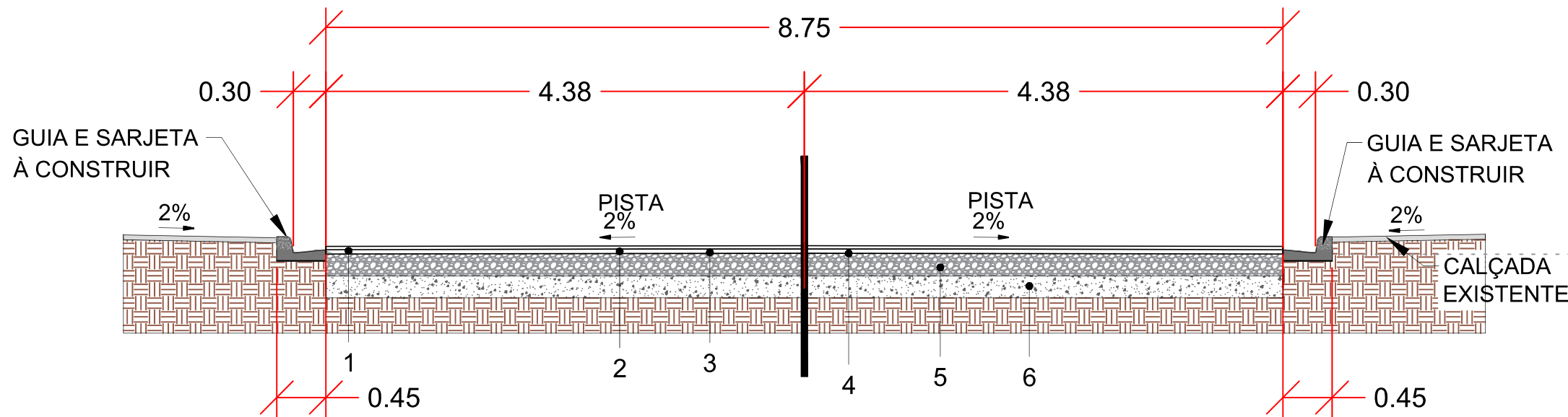
CORTE TRANSVERSAL A-A RECUPERAÇÃO DE BASE PARA PAVIMENTAÇÃO ASFÁLTICA COM CBUQ RUA DENISE ESC. 1:50
