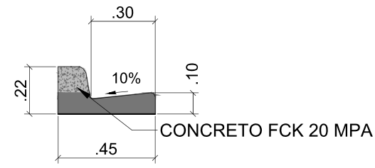
DETALHE GUIA E SARJETA EXTRUSADA ESC 1/25. - MEDIDAS EM M
