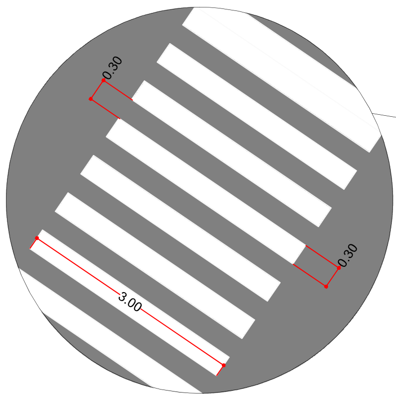
DET. FAIXA DE PEDESTRES Sem escala
