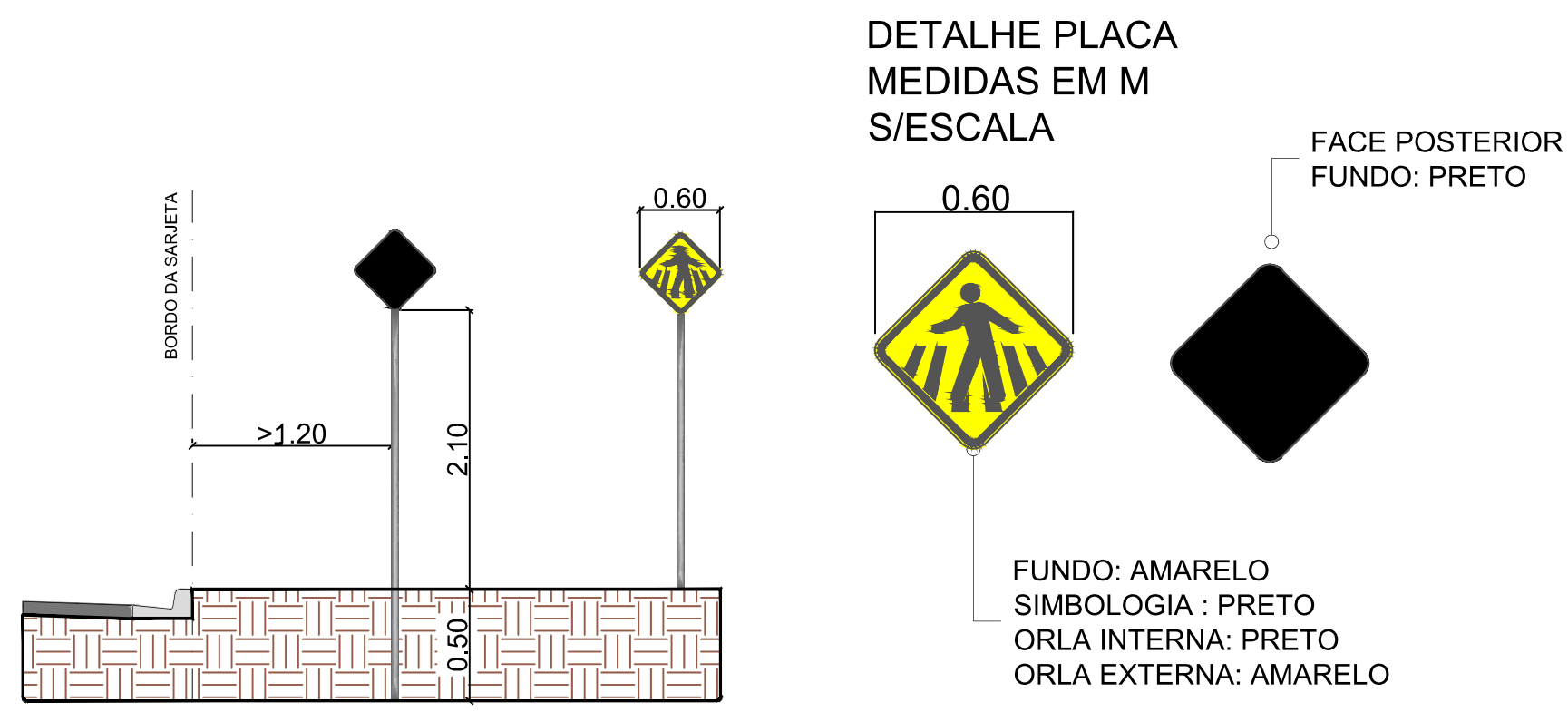
DETALHE PLACA A32b PASSAGEM SINALIZADA DE PEDESTRES PLACA - ELEVÇÃO MEDIDAS EM M S/ESCALA
