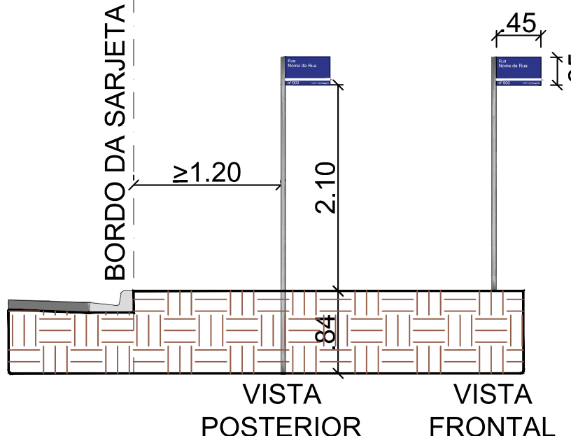
DETALHE PLACA LOGRADOURO PLACA - ELEVACÃO MEDIDAS EM M S/ESCALA
