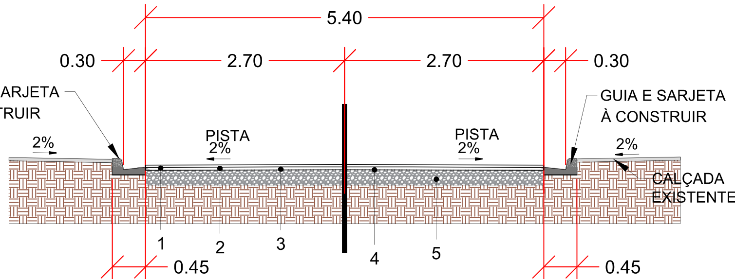
CORTE TRANSVERSAL B-B PAVIMENTAÇÃO ASFÁLTICA COM CBUQ RUA KALLIL SELEM SAFADI ESC. 1:50
