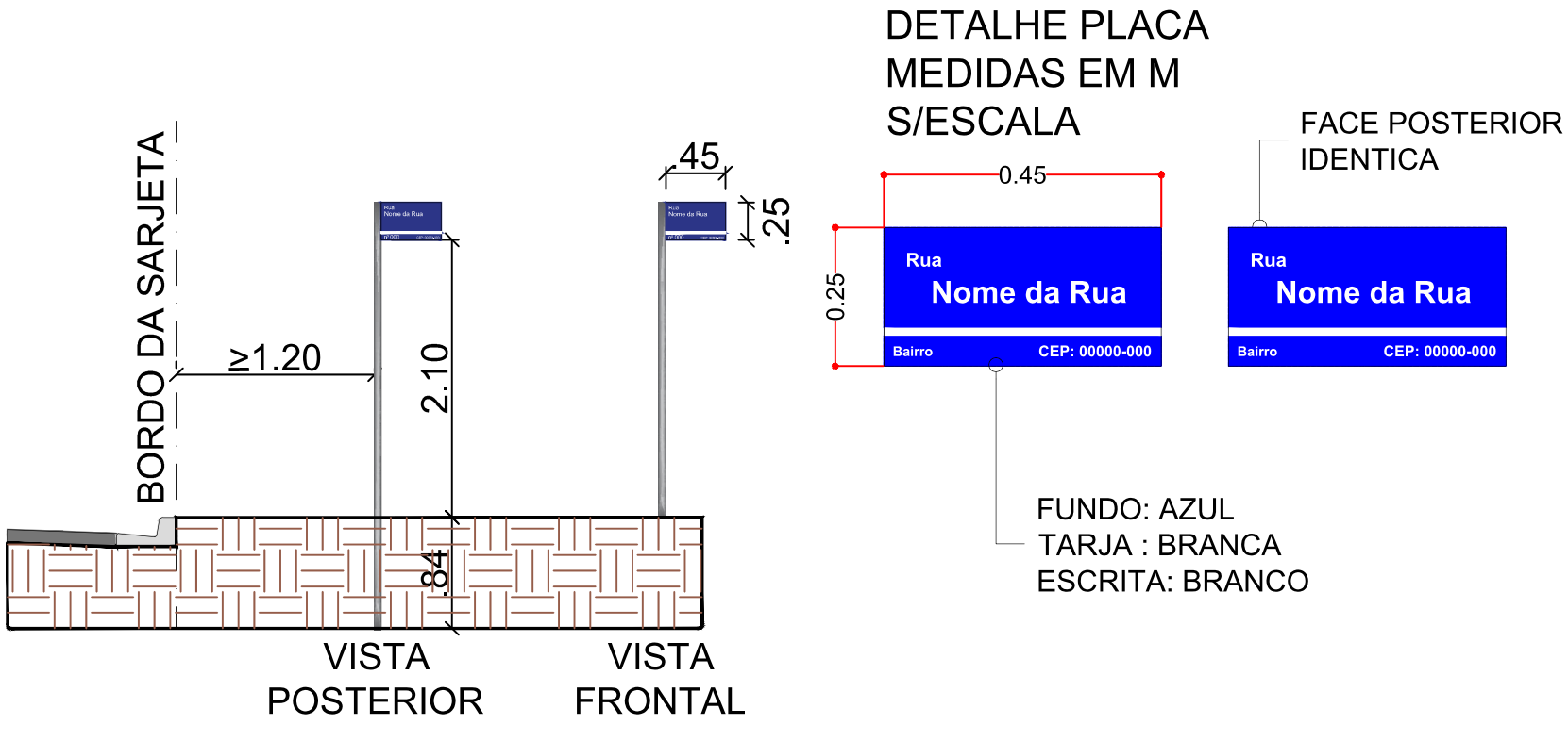
DETALHE PLACA LOGRADOURO PLACA - ELEVÇÃO MEDIDAS EM M S/ESCALA
