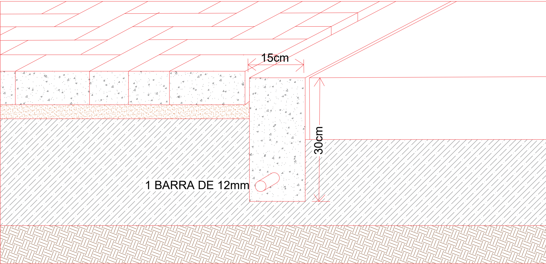
DETALHE VIGA DE CONTENÇÃO SITUAÇÃO S/ESCALA
