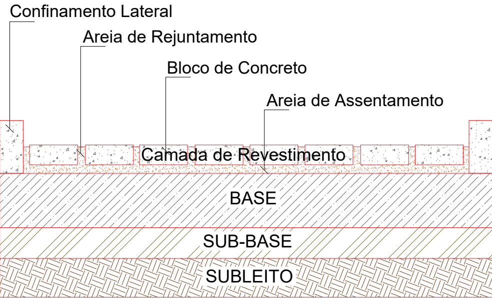
DETALHE RECAPEAMENTO SITUAÇÃO S/ESCALA
