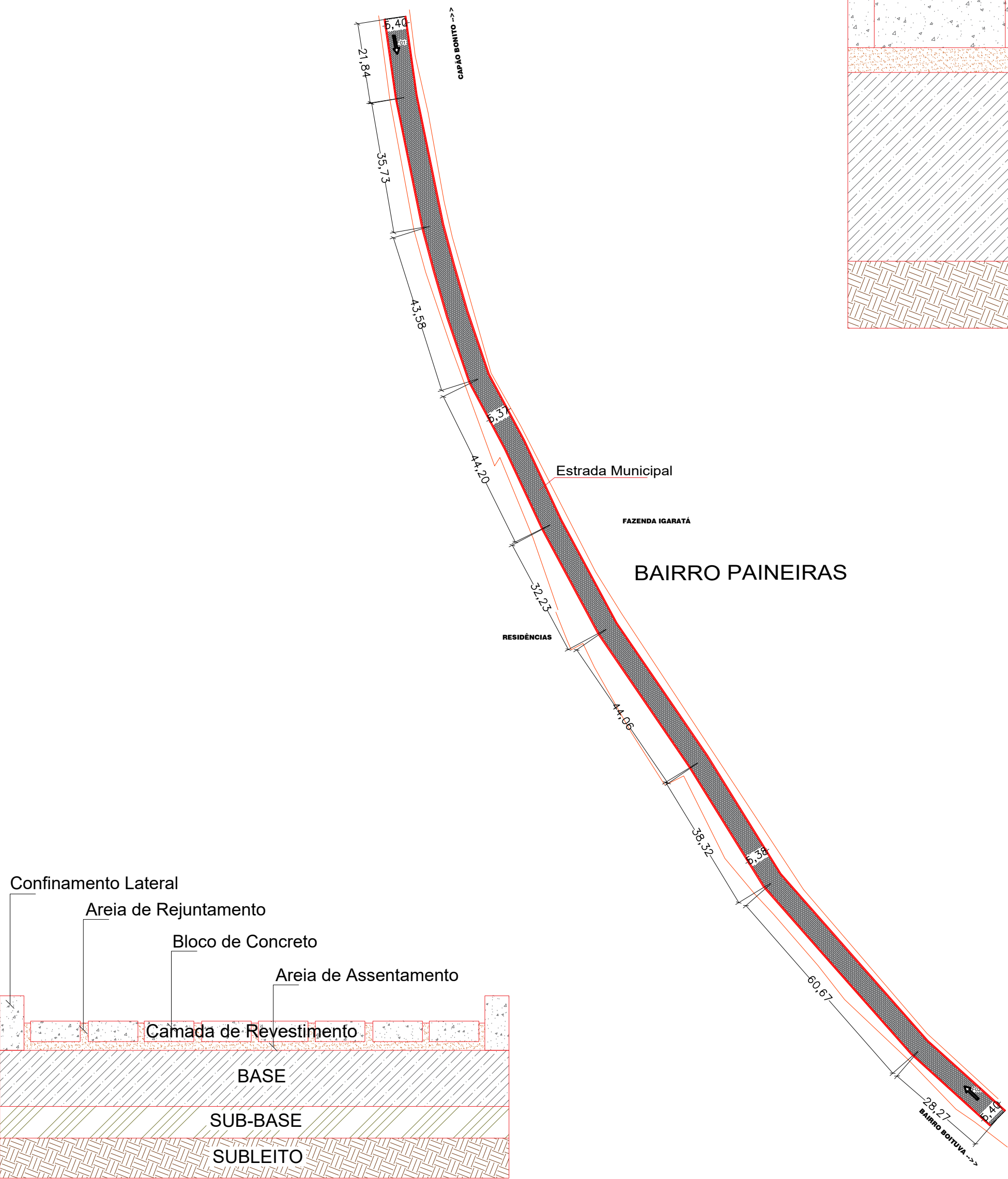
DETALHE RECAPEAMENTO SITUAÇÃO S/ESCALA
