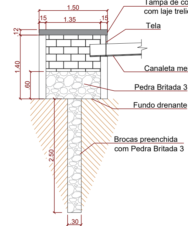
CAIXA DRENANTE CORTE AA esc 1:50
