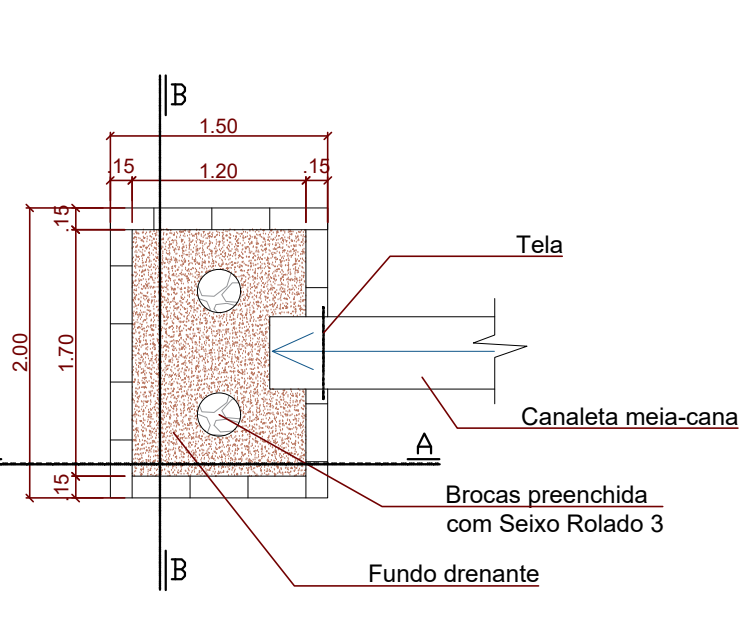
CAIXA DRENANTE PLANTA BAIXA esc 1:50
