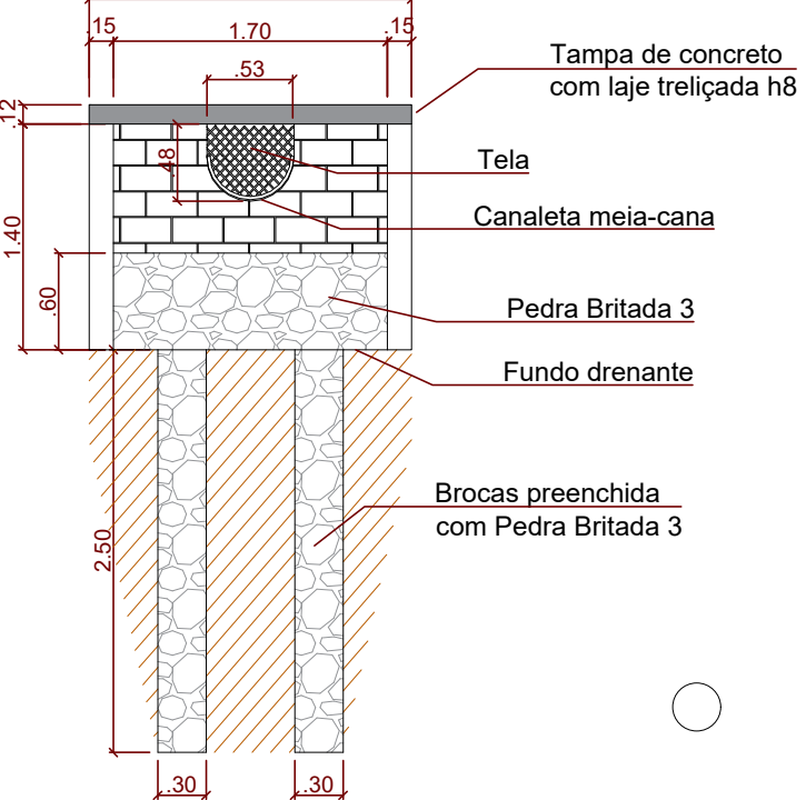
CAIXA DRENANTE CORTE BB esc 1:50
