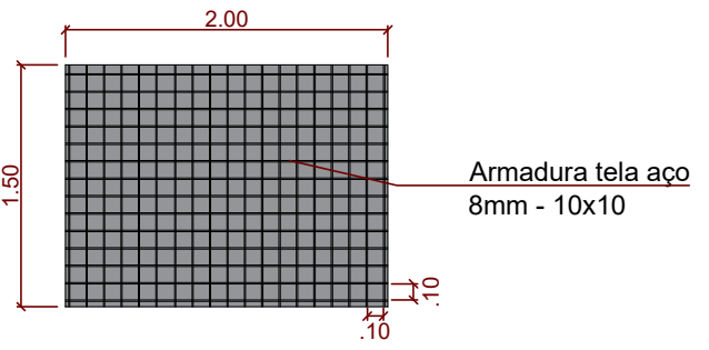
PLANTA BAIXA TAMPA CONCRETO esc 1:50
