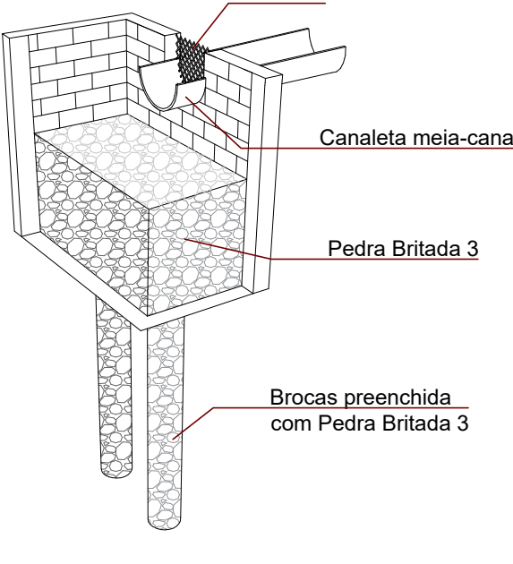
CAIXA DRENANTE PERSPECTIVA esc 1:50
