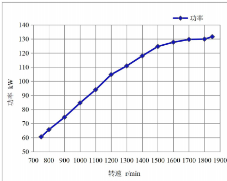
Curva de variação de potência com rotação do motor
