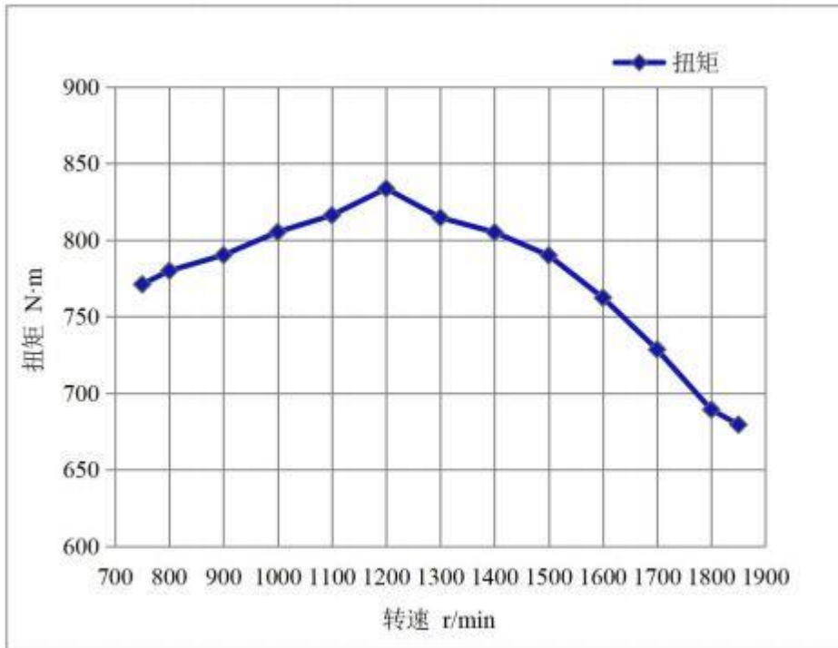
Curva de variação de torque com rotação do motor
