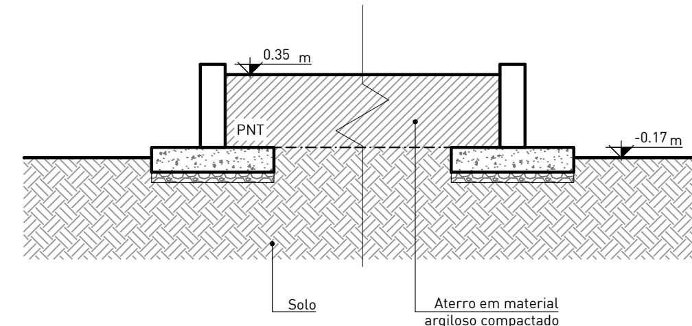
03 CAIXOTE CORTE ESCALA 1:25
