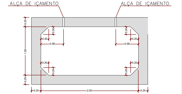
SEÇÃO ADUELA s/escala
