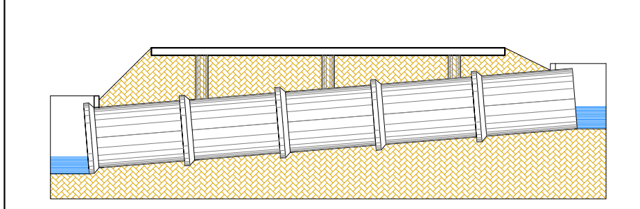
DETALHE BOCA DE LOBO
