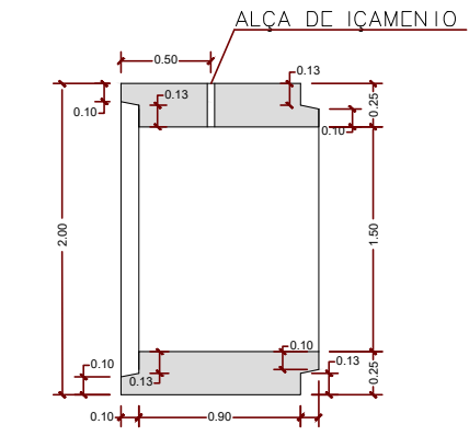
CORTE ADUELA s/escala
