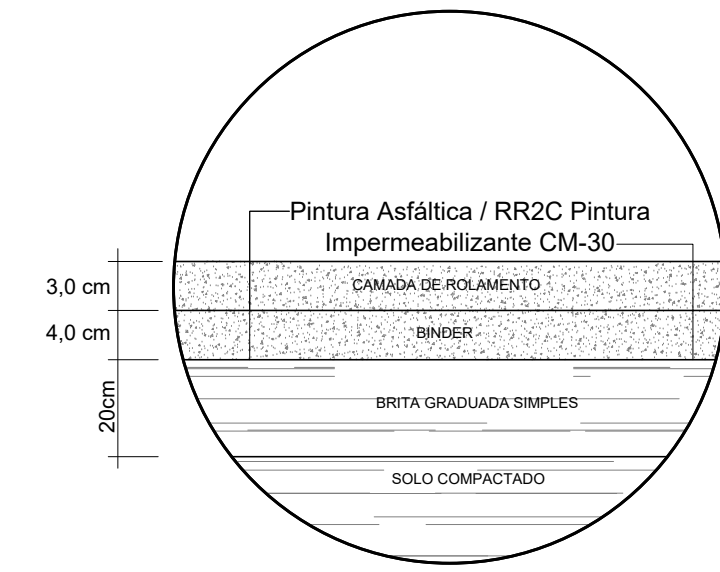
DETALHE PAVIMENTAÇÃO SITUÇÃO S/ESCALA
