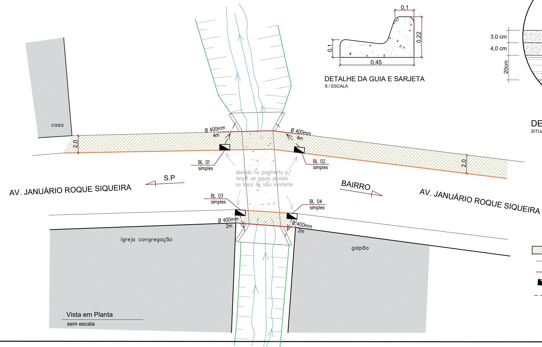
DETALHE BOCA DE LOBO
