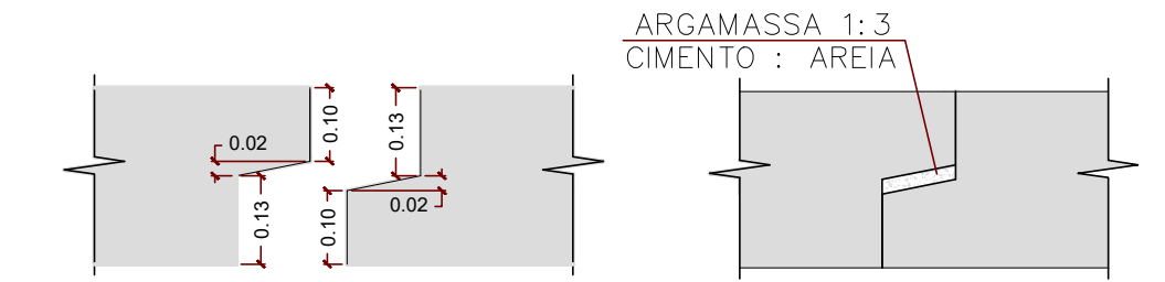
DETALHE ASSENTAMENTO s/escala
