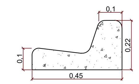
DETALHE DA GUIA E SARGETA S/ESCALA
