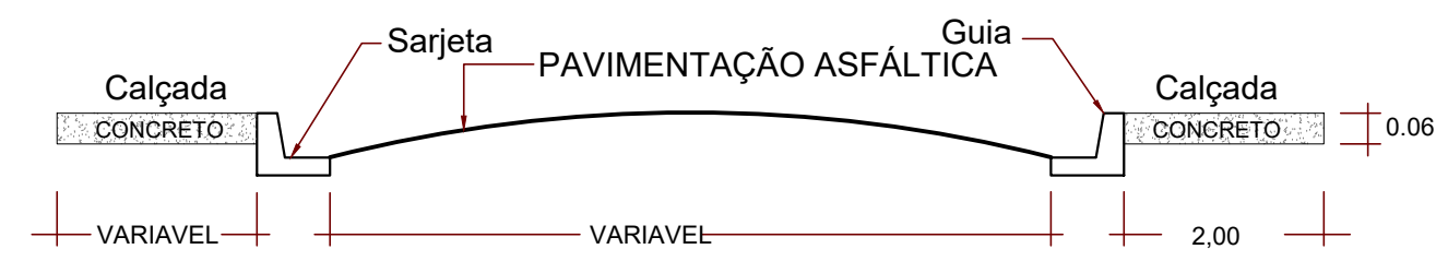
PERFIL A.A TRANSVERSAL DO LEITO DAS RUAS S/ESCALA
