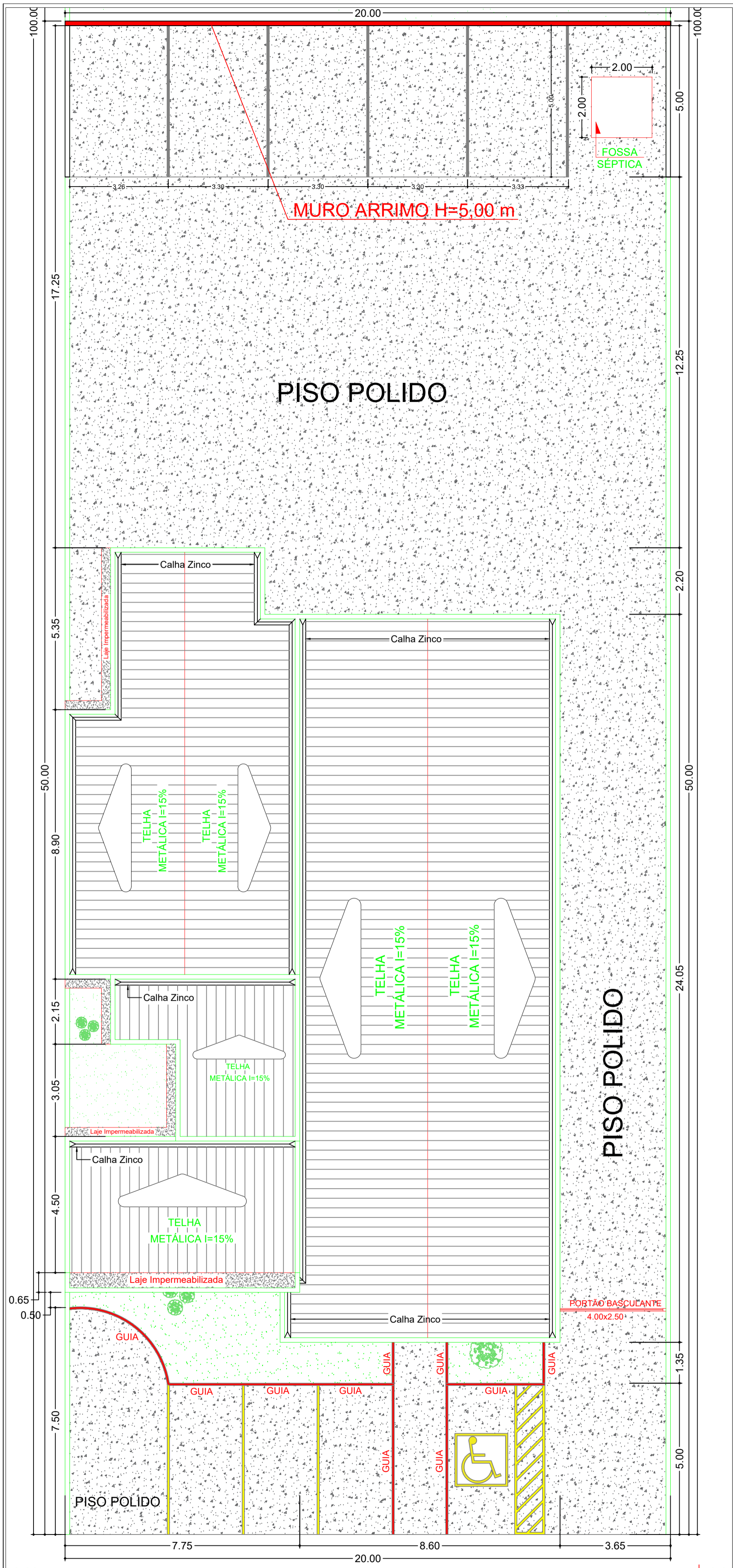
Calçada = 3.00m EXECUÇÃO DE PISO EXTERNO/GUIA/JARDIM ESCALA 1/100
