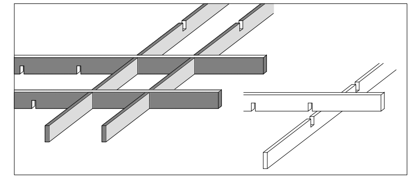
DETALHE TRAVAMENTO PERGOLADO
